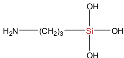
3-Aminopropylsilanetriol
